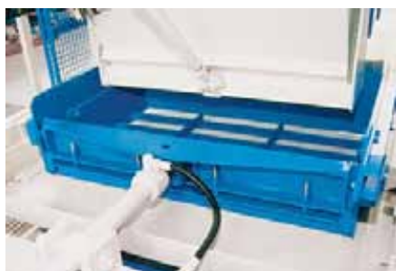
Гидропривод трансферкары
